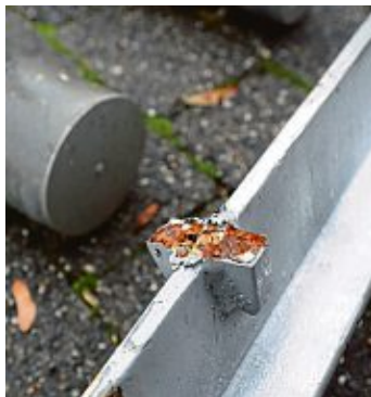
Rost hat sich durch die Stahlkonstruktion gefressen.
