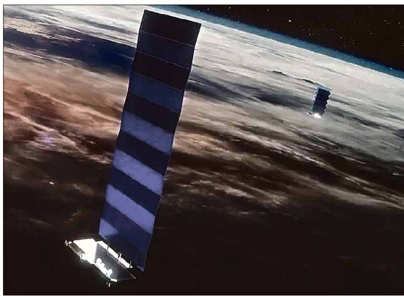
Die kleinen Starlink-Satelliten reflektieren die Sonne und leuchten am Himmel.
