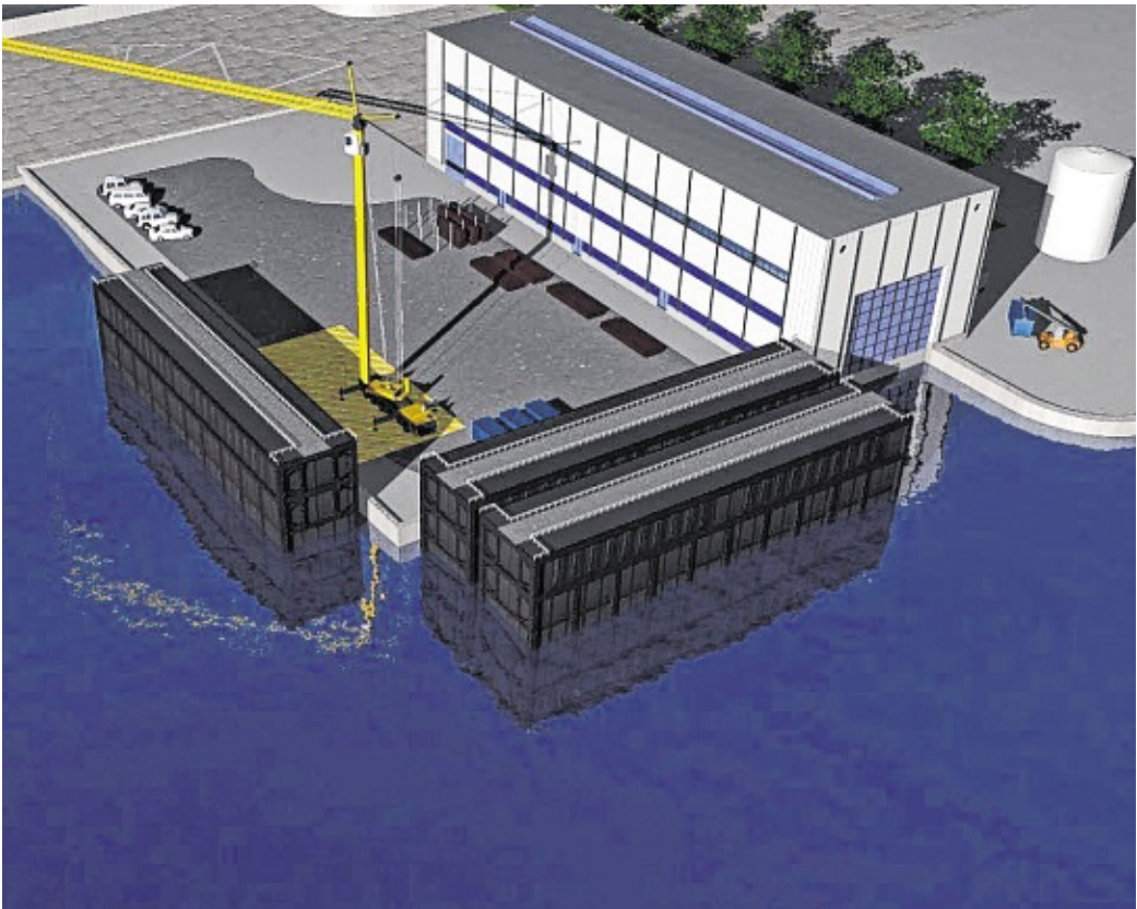
Das Trockendock soll am WSA-Betriebshafen an der Ostermoorer Straße errichtet werden In der Grafik sind drei Schleusentore dort geparkt. GRAFIK: WSA BRUNSBÜTTEL,
