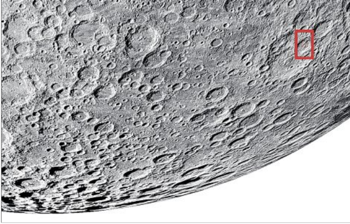
Der Krater Fabricius (roter Rahmen) liegt in der Nähe des Mondsüdpols (links unten).
