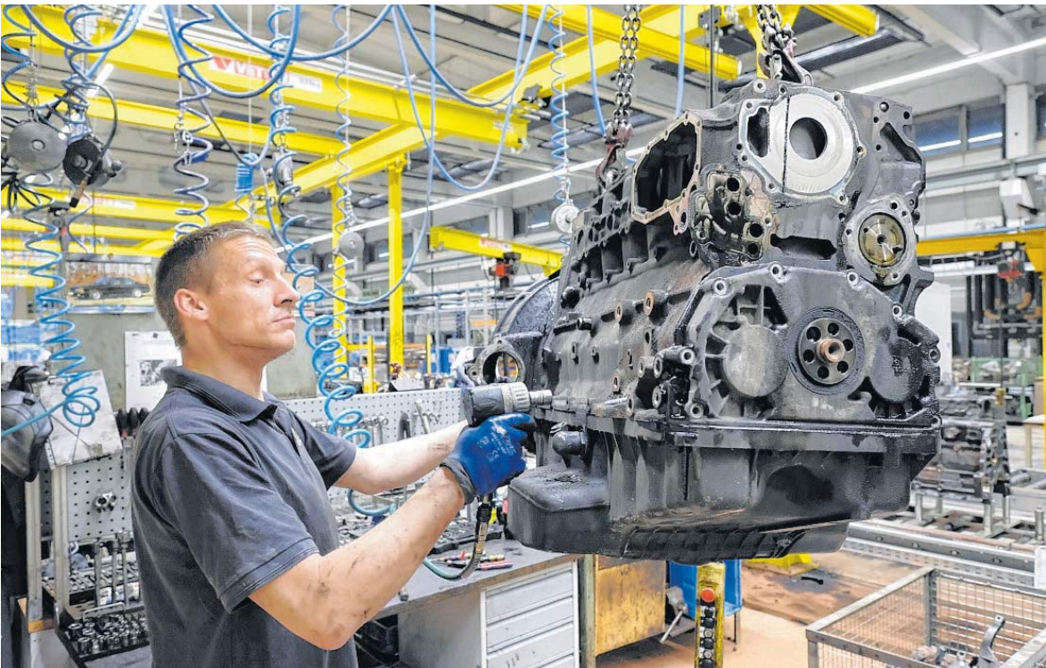
David Häußer bei der Demontage eines Diesellaggregats in den Wolfswerken Sachsen in Wolfspfütz. Rund 4000 gebrauchte Motoren werden hier pro Jahr industriell aufbereitet.
