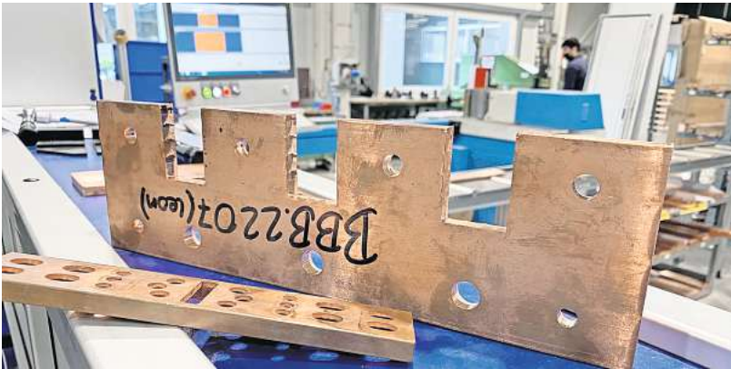
Für die Schaltschränke müssen auch Kupferteile ausgestanzt werden.
